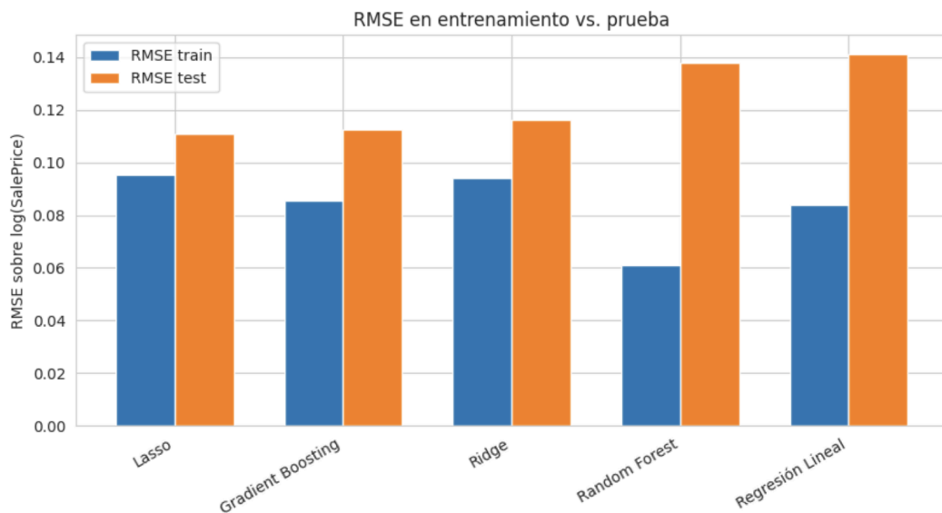
Fig. 5. Comparativa de Modelos
